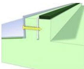
Bild 2: Optimaler unterer Fensteranschluss mit dem PR003 Fensterbankformteil: schlagregendicht, wärmedämmend, luftdicht
