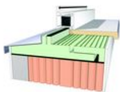
Bild 1: Zusätzliche mechanische Befestigung der Außenfensterbank mittels einer PVC-Leiste und einer Schraube
